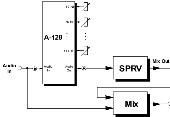
Abb. 2: frequenzselektiver Hall
